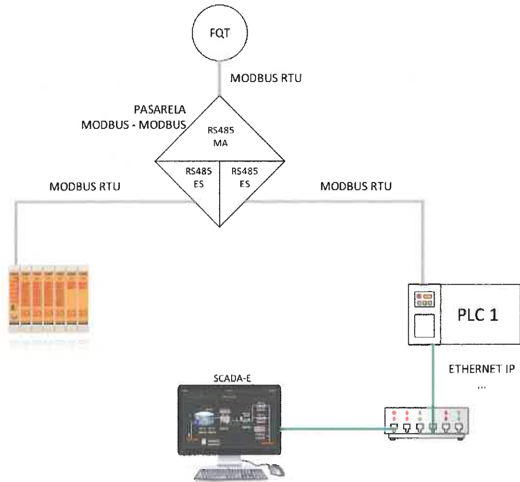
Ejemplo de conexión con caudalímetro mediante pasarela MODBUS
