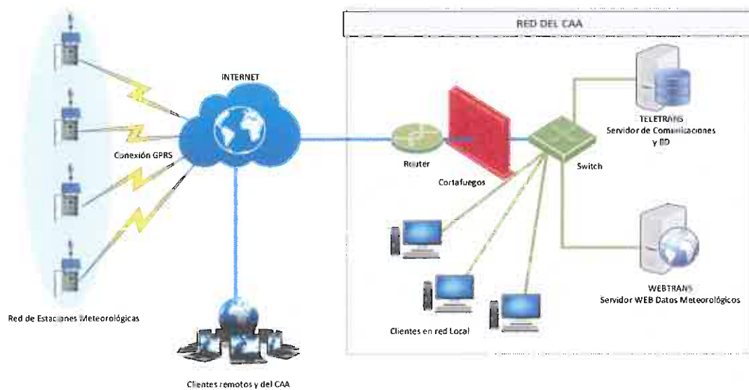
Esquema de red de estaciones meteorológicas
