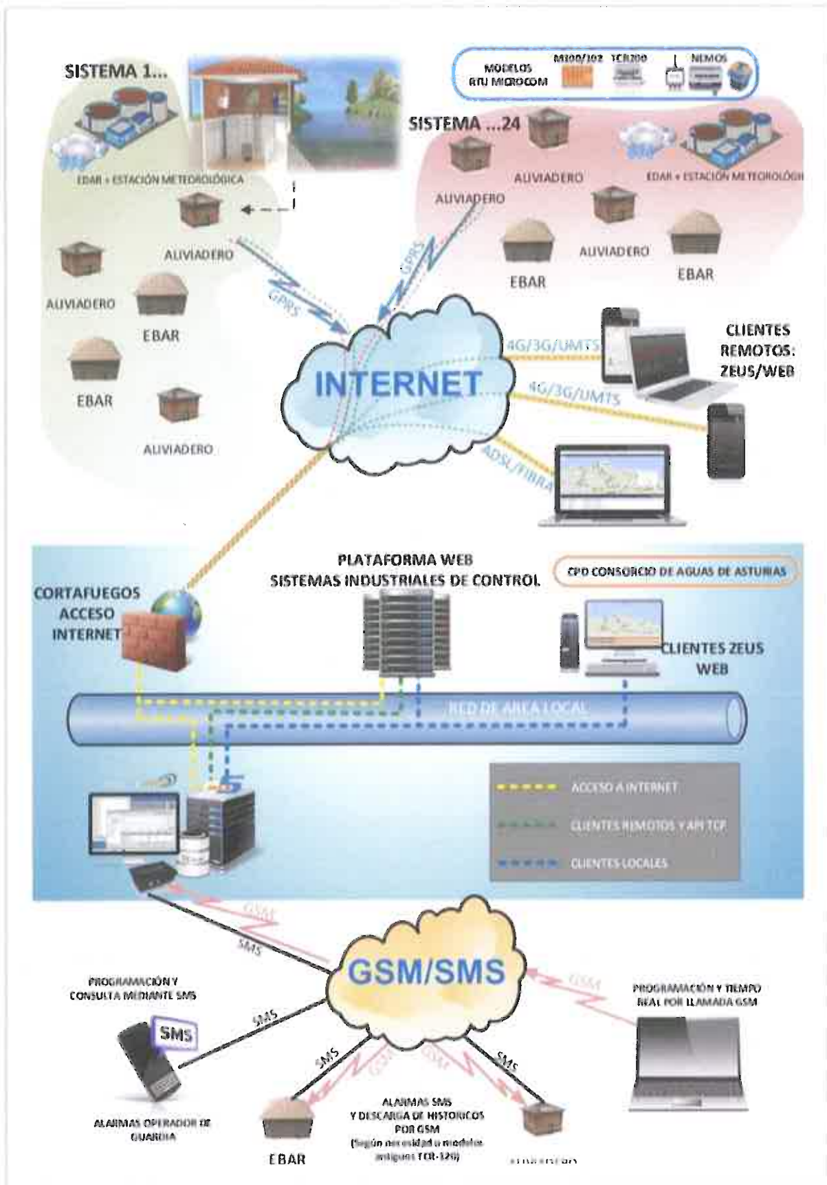
Esquema general de comunicaciones del centro ZEUS5 WEB en el Centro de Datos
