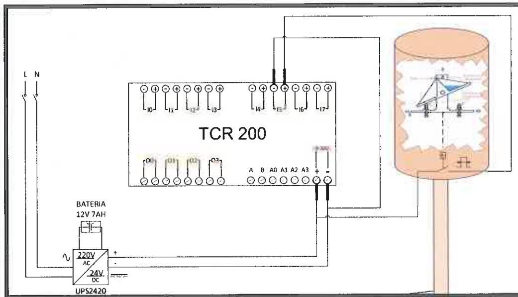
Ejemplo de conexión de pluviómetro a equipo de telemetría
