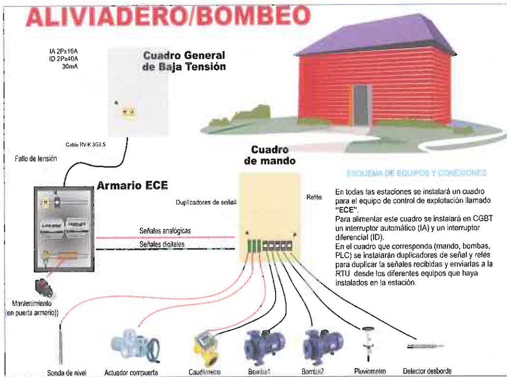
Esquema básico de conexiones de una estación.
